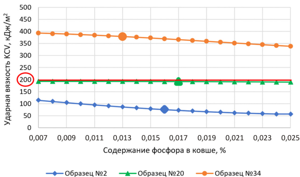
Рис. 4. Зависимость прогнозируемой ударной вязкости образцов-свидетелей от параметра «Содержание фосфора в ковше»
