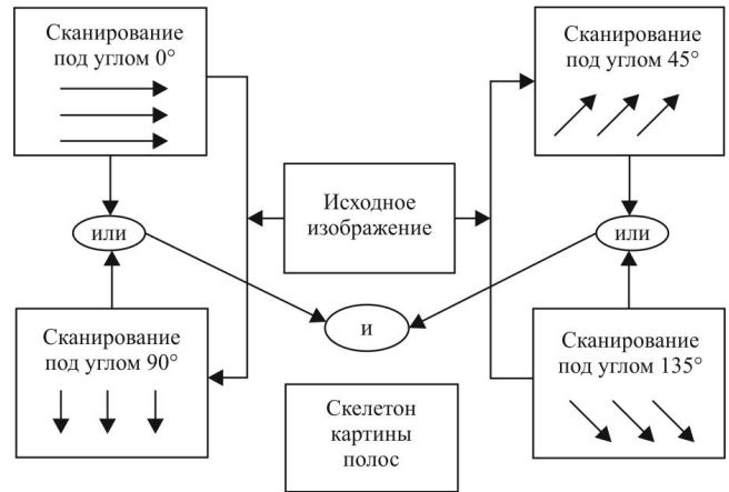
Рис. 6. Общий вид алгоритма построения скелетона изображения изохроматических полос
