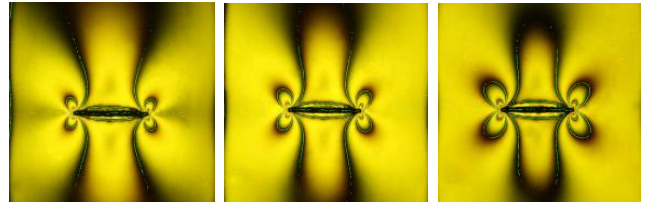
Рис. 7. Результаты цифровой обработки экспериментальной информации
