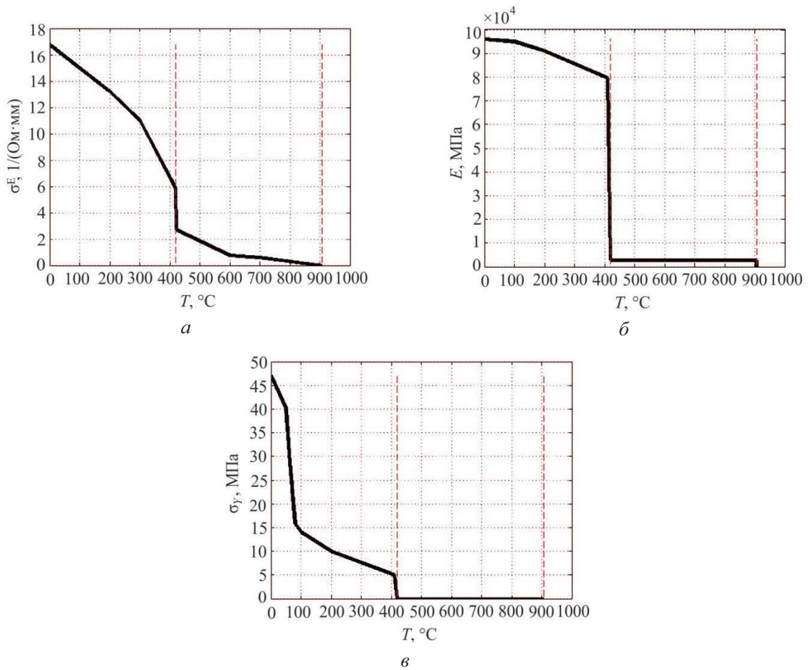
Рис. 2. Зависимости (а) электропроводности \sigma^E ; (б) модуля Юнга E ; (в) предела текучести \sigma_\gamma от температуры T (вертикальными штриховыми линиями отмечены температуры плавления T_{melt} = 419^\circ C и испарения T_{evap} = 906^\circ C )
