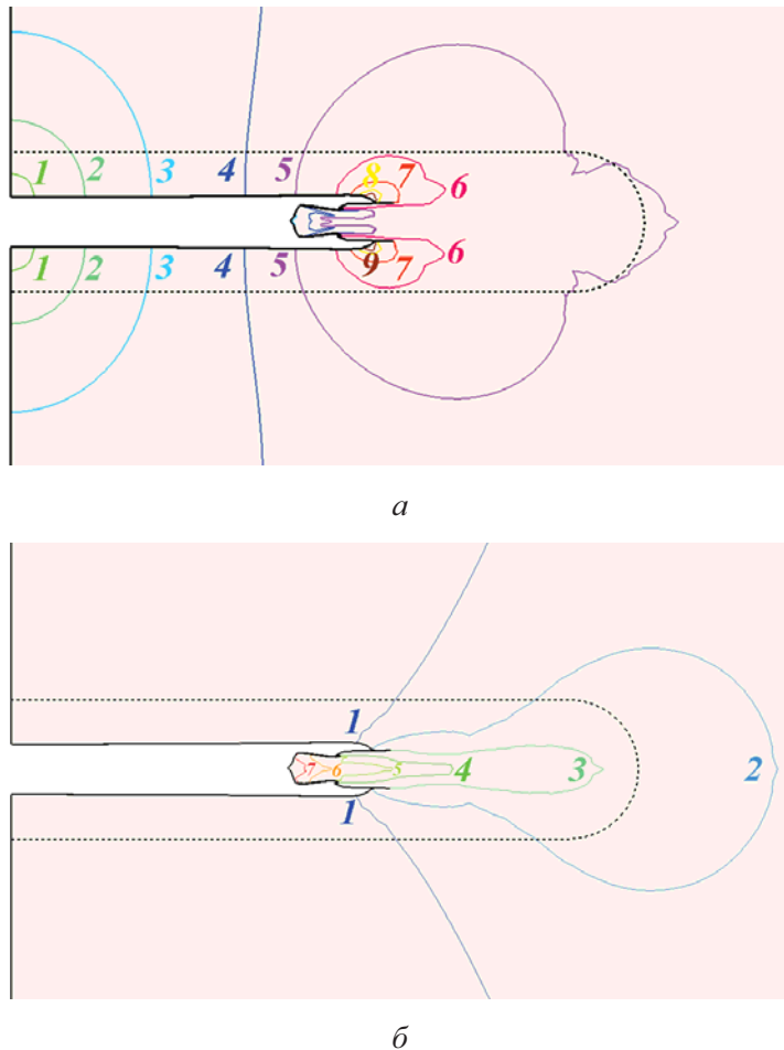
Рис. 4. Изолинии (а) плотности тока A/mm^2 и (б) температуры ^{\circ}C при t = 24,5 мкс в окрестности микротрещины. Начальная температура 20 ^{\circ}C , приложенный ток 7,3 kA/mm^2 ; а – распределение плотности электрического тока A/mm^2 : 1 – 500, 2 – 1500, 3 – 3000, 4 – 6000, 5 – 9000, 6 – 15000, 7 – 21000, 8 – 27000, 9 – 30000; б – распределение температуры ^{\circ}C : 1 – 50, 2 – 100, 3 – 200, 4 – 300, 5 – 350, 6 – 400, 7 – 419
