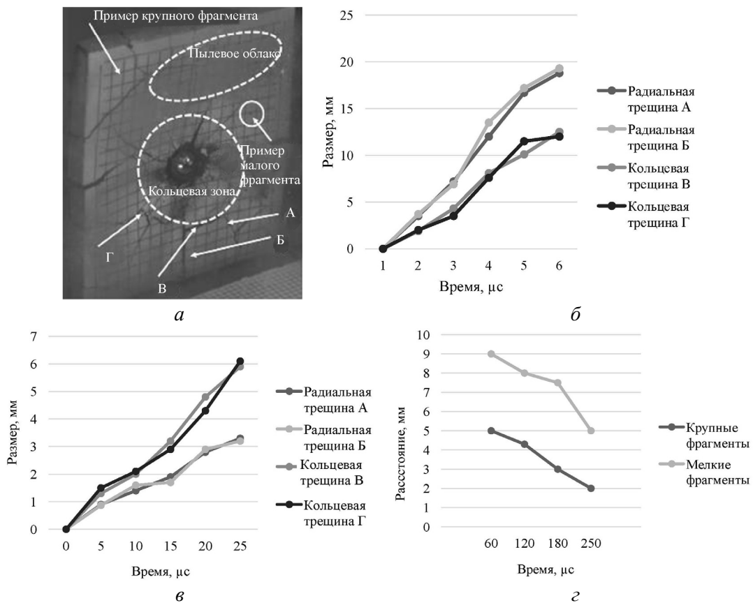
Рис. 5. Визуализация процессов фрагментации мишени из синтетического минерального сплава на основе горнблендита и результаты расчета ее параметров: а – наблюдаемые явления и объекты, характеризующие фрагментацию; б – скорость роста радиальных и кольцевых трещин; в – скорость увеличения толщины трещин; г – динамика скорости фрагментов мишени разного размера
