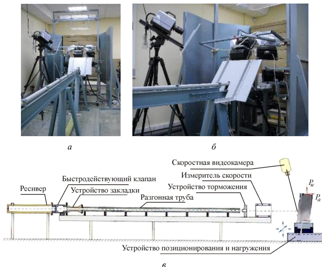
Рис. 1. Экспериментальный комплекс: а – вид со стороны разгонной трубы; б – камера с образцом и оборудованием для видеофиксации; в – схема установки
