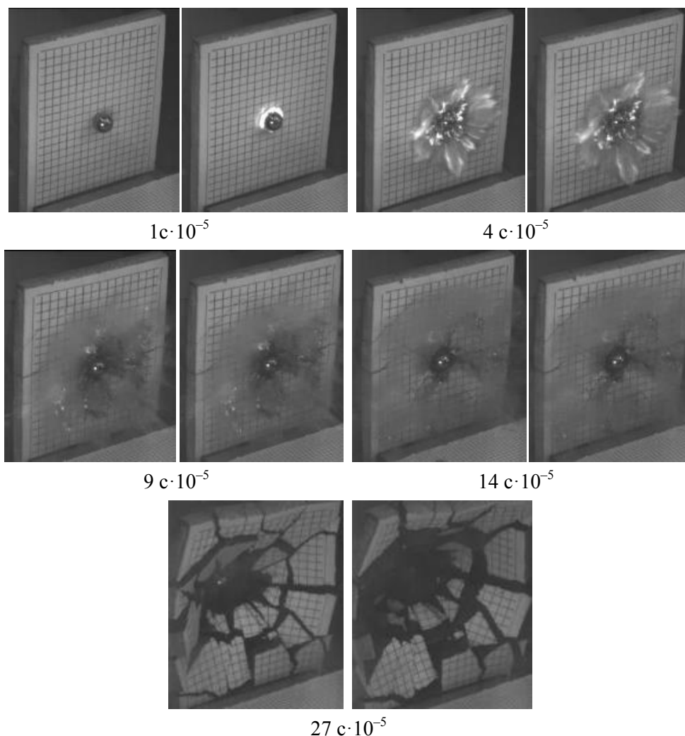
Рис. 3. Фреймовая карта высокоскоростной съемки разрушения образца синтетического минерального сплава на основе горнблендита при скорости 233 м/с
