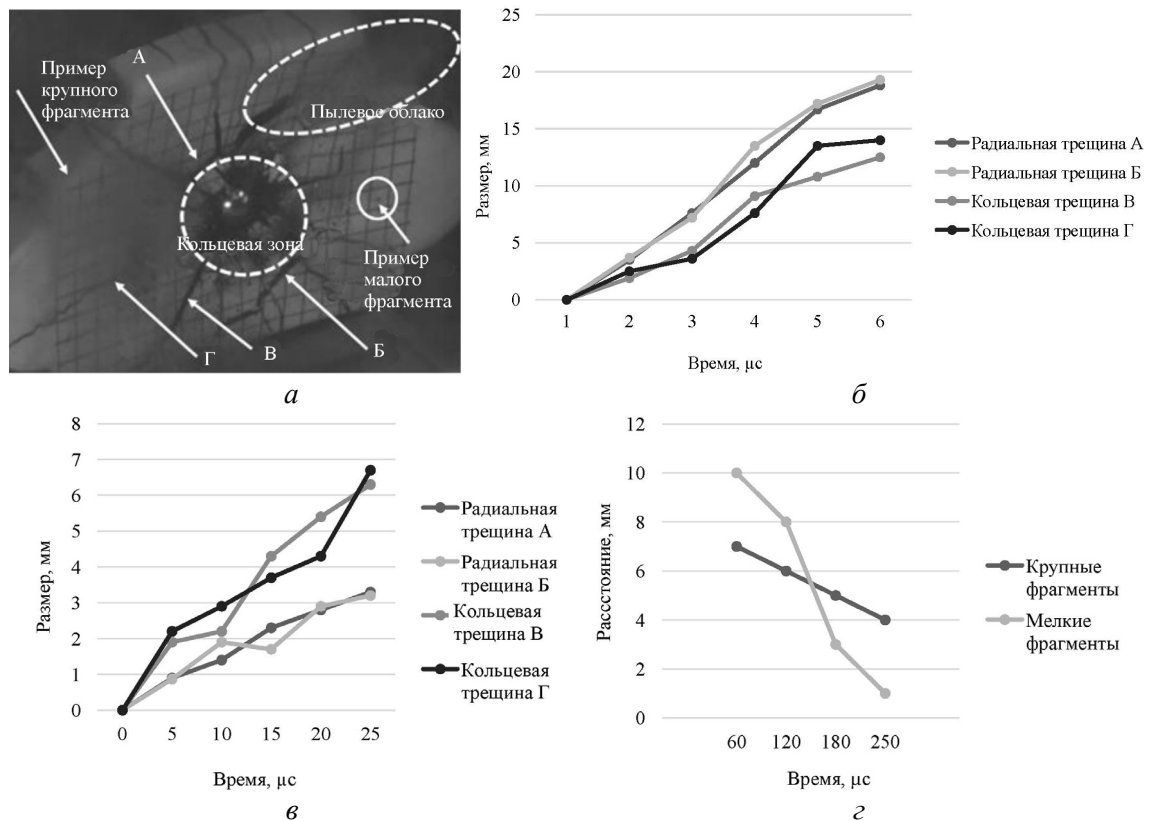
Рис. 6. Визуализация процессов фрагментации мишени из синтетического минерального сплава на основе базальта и результаты расчета ее параметров: а – наблюдаемые явления и объекты, характеризующие фрагментацию; б – скорость роста радиальных и кольцевых трещин; в – скорость увеличения толщины трещин; г – динамика скорости фрагментов мишени разного размера
