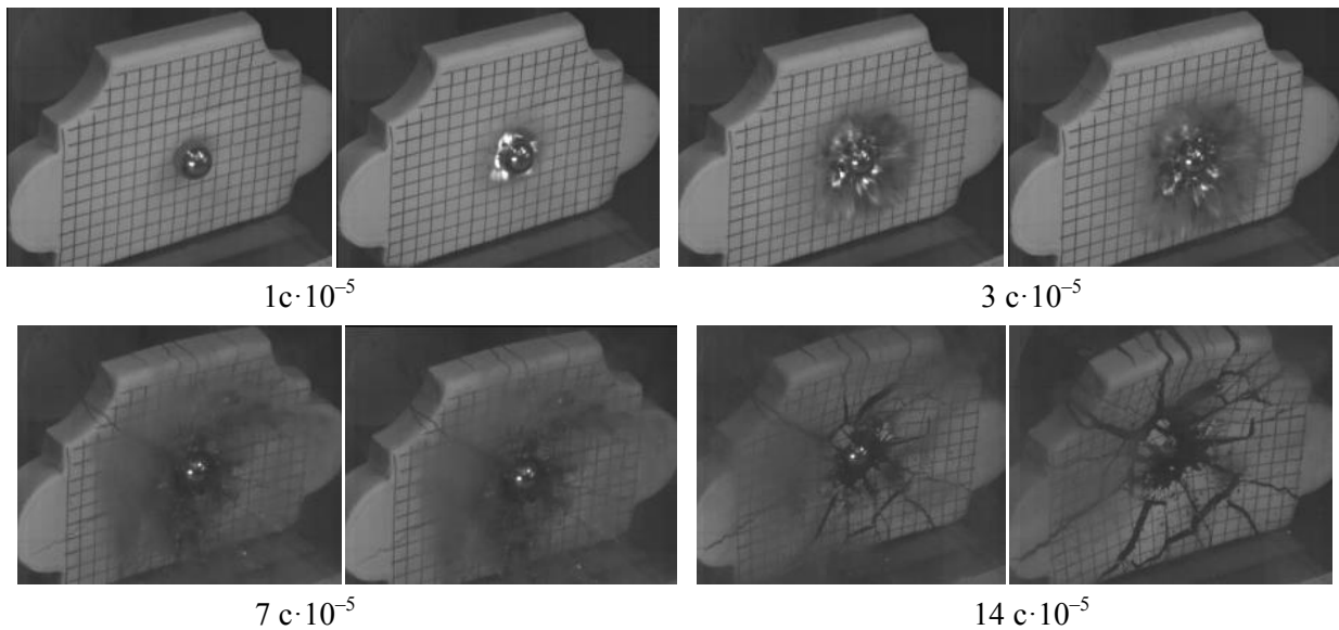
Рис. 4. Фреймовая карта высокоскоростной съемки разрушения образца синтетического минерального сплава на основе базальта при скорости 234 м/с
