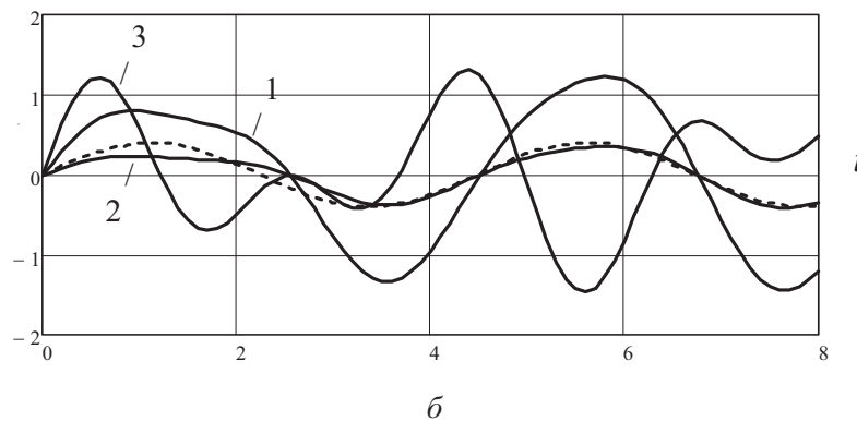
Рис. Графики изменения W(r, \theta, z, t) и Q(t) во времени: a - \mu = 0,2\lambda_{imn} (i, n, m = 1) ; b - \mu = 0,7\lambda_{imn} (i, n, m = 1) ; 1 – W(1, \pi/2, 0, t) ; 2 – W(1, 3\pi/2, 0, t) ; 3 – Q(t)
