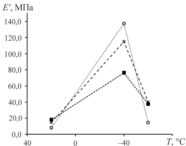
Рис. 3. Графики зависимостей динамических модулей упругости полиуретана от температуры: x- МДИ; ■- ТДИ; o- НДИ
