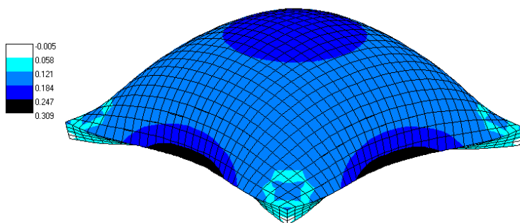
Рис. 3. Распределение интенсивности пластических деформаций
