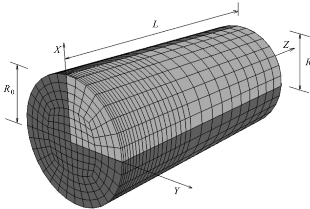
Рис. 1. Конечно-элементная дискретизация половины стержня
