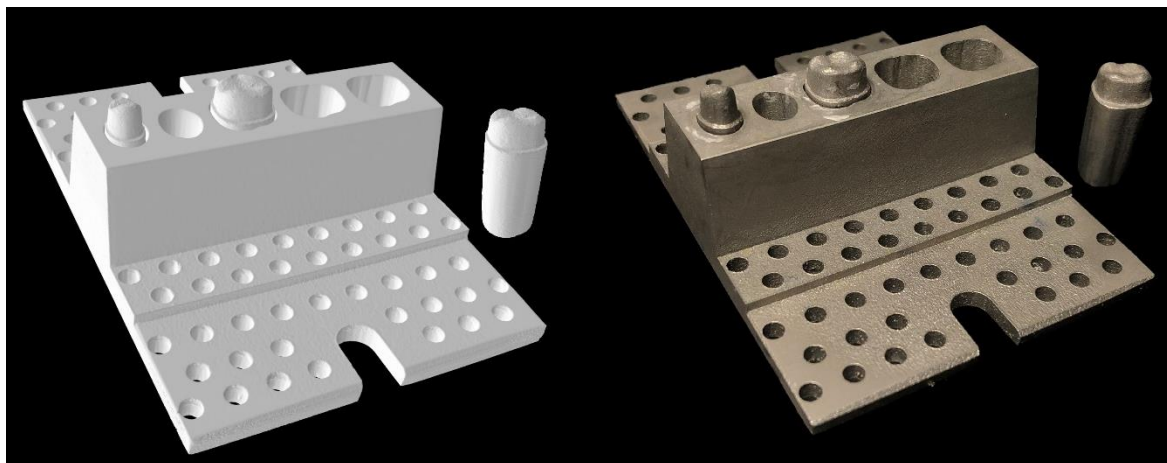
Рис. 1. Универсальная оснастка для экспериментального исследования прочностных характеристик адгезивного мостовидного протеза разной протяженности: a – компьютерная модель; б – стальная оснастка, изготовленная с помощью 3D-печати
